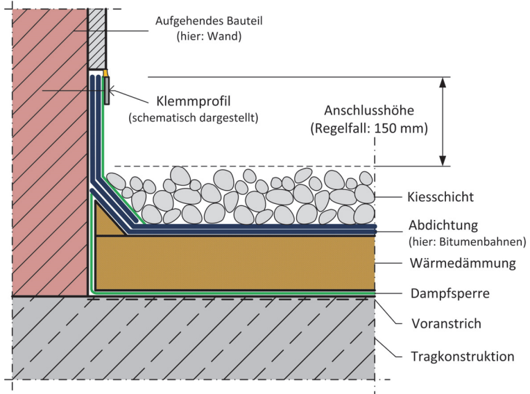
Bild 65: Keil am Übergang von Dachfläche und aufgehendem Bauteil bei Abdichtungen mit Bitumenbahnen sowie Definition der Anschlusshöhe (Quelle: Schmidt)
